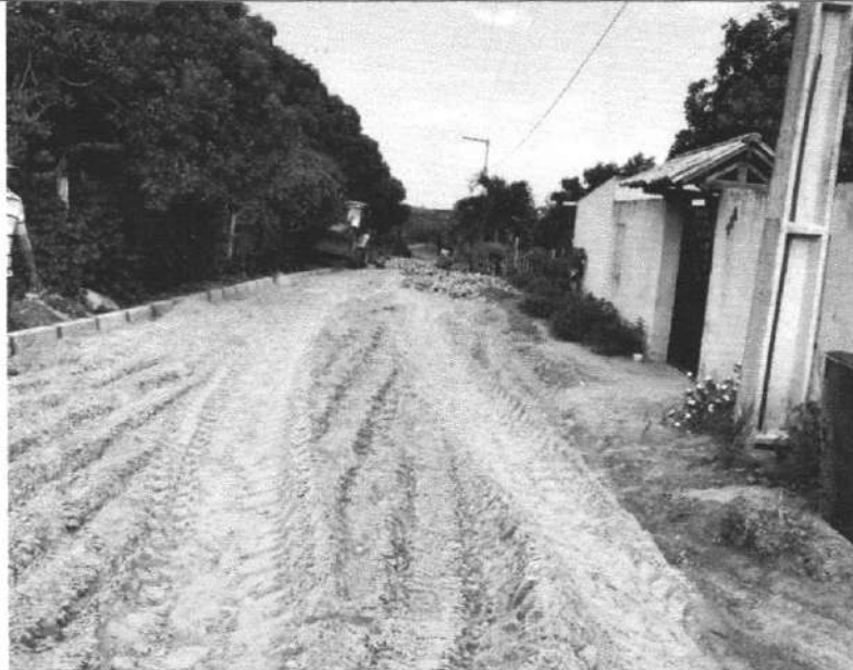
RUA C - ATERRO COM AREIA FINA, COMPACTADO MECANICAMENTE, INCLUSIVE AQUISIÇÃO EM DEPÓSITO DE MATERIAL | TRANSPORTE COM CAMINHÃO BASCULANTE DE 14 M³
