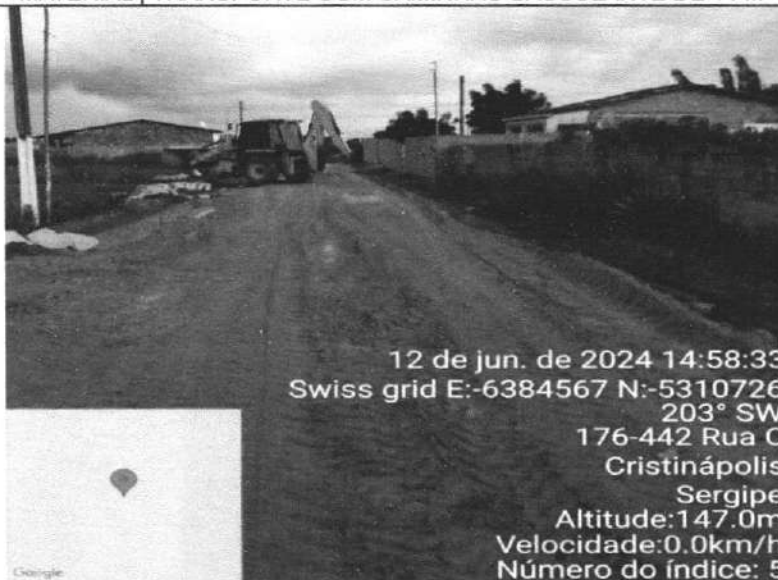
RUA C - ATERRO COM AREIA FINA, COMPACTADO MECANICAMENTE, INCLUSIVE AQUISIÇÃO EM DEPÓSITO DE MATERIAL | TRANSPORTE COM CAMINHÃO BASCULANTE DE 14 M 3
