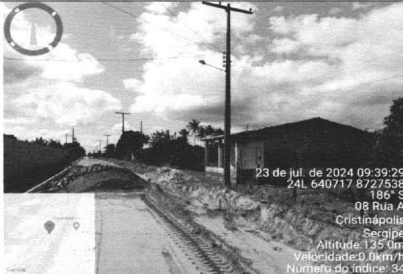
RUA A - ATERRO COM AREIA FINA, COMPACTADO MECANICAMENTE, INCLUSIVE AQUISIÇÃO EM DEPÓSITO DE MATERIAL | TRANSPORTE COM CAMINHÃO BASCULANTE DE 14 M 3
