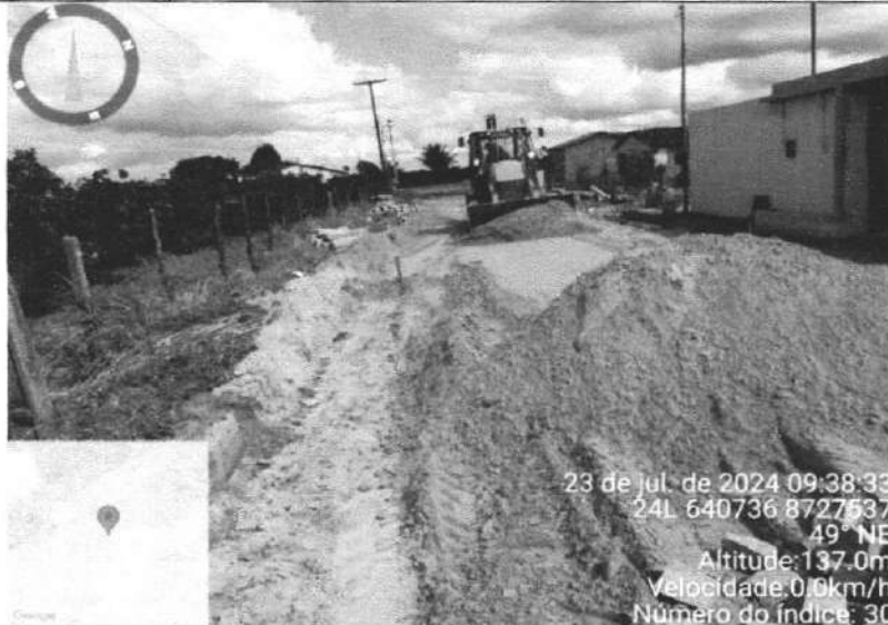
ATERRO COM AREIA FINA, COMPACTADO MECANICAMENTE, INCLUSIVE AQUISIÇÃO EM DEPÓSITO DE MATERIAL | TRANSPORTE COM CAMINHÃO BASCULANTE DE 14 M³
